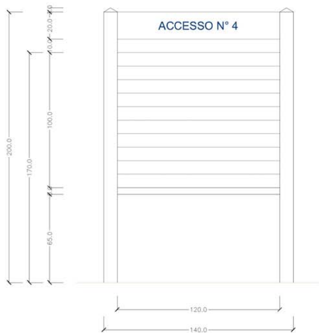
PROSPETTO
