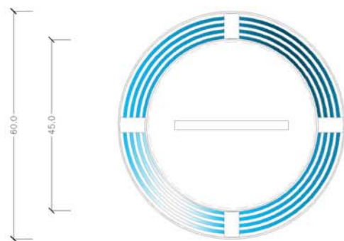
PROSPETTO
