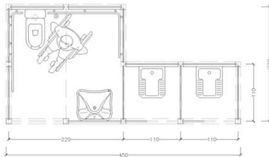
PIANTA
