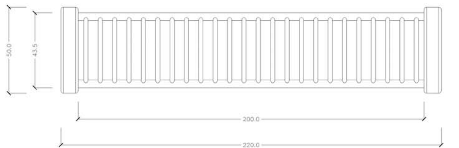
PIANTA
