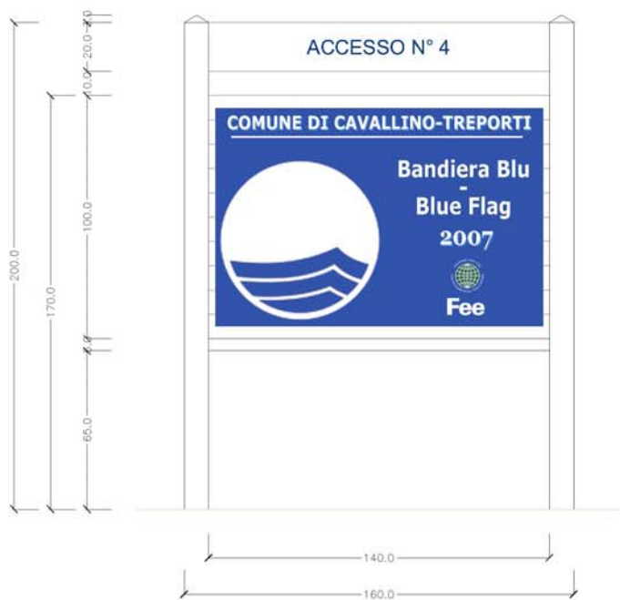
PROSPETTO
